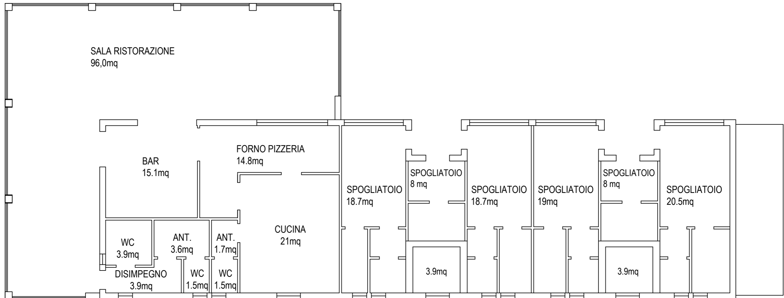
PLANIMETRIA STATO DI FATTO ALLA DATA DEL 9.04.2026_scala 1:100
